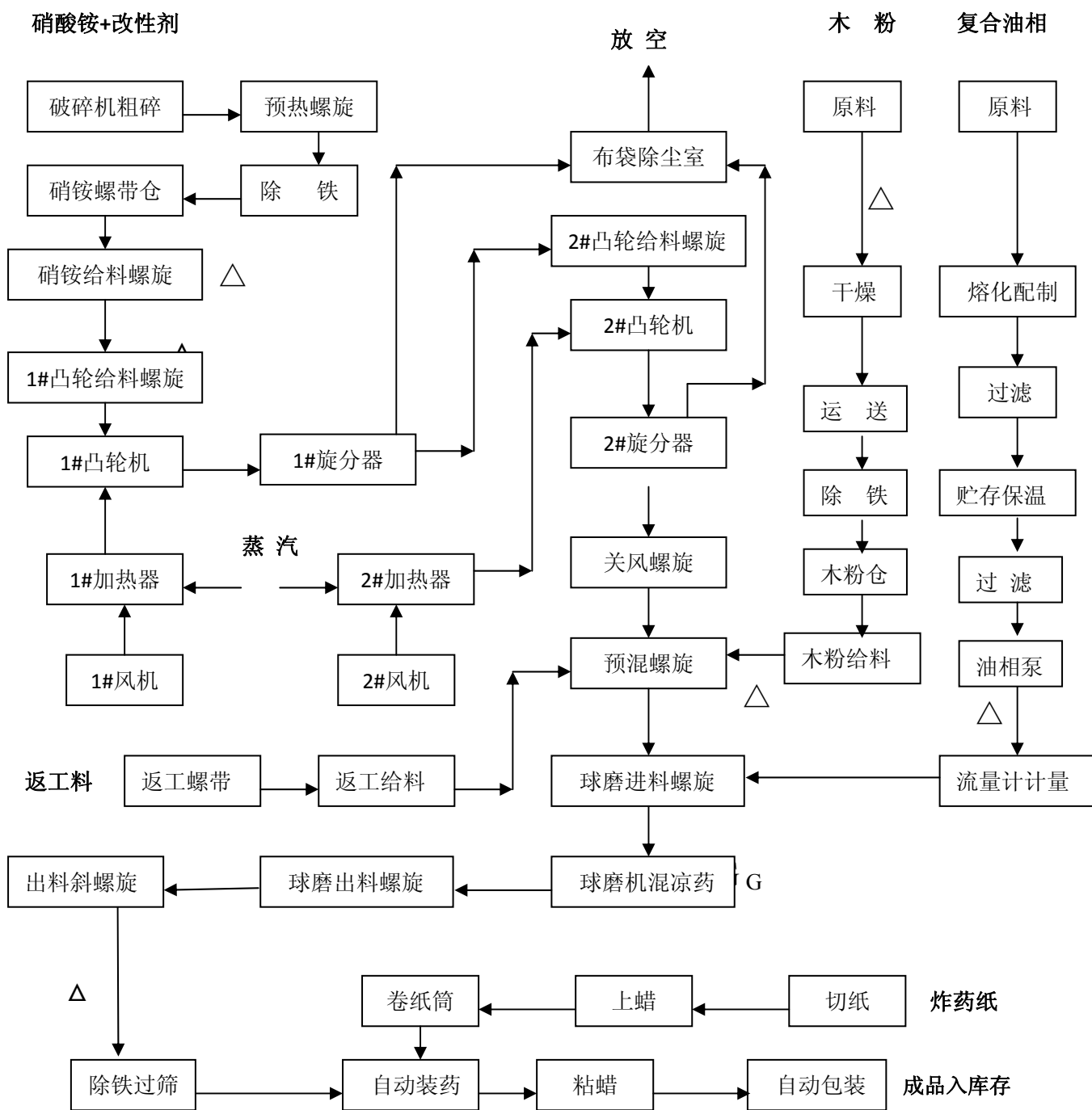
改性铵油炸药连续化自动化生产线工艺流程图
