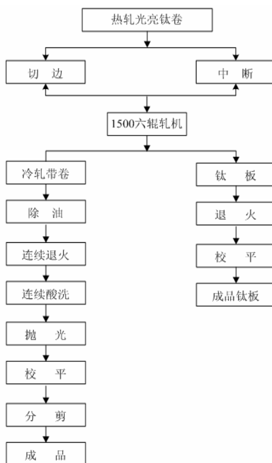
冷轧钛材生产工艺流程图
