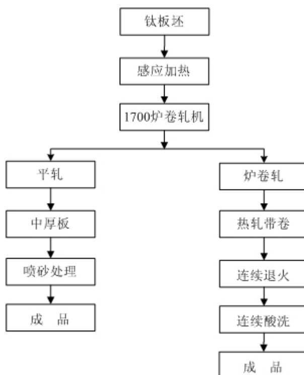
热轧板材生产工艺流程图
