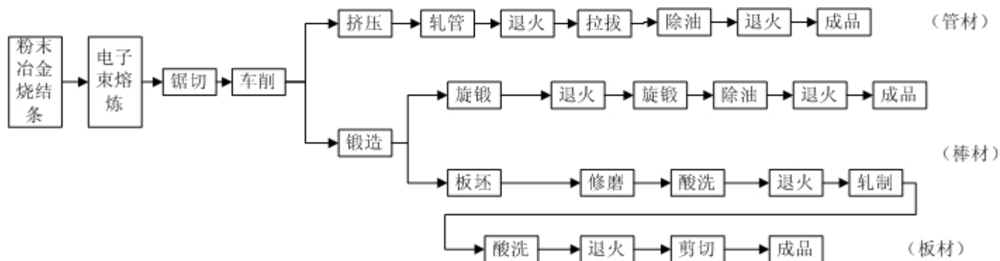
钽铌制品工艺流程图
