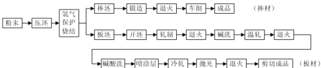
钽铌制品工艺流程图
