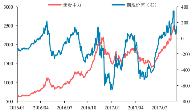
图 10：焦炭期现价差 单位：元/吨
