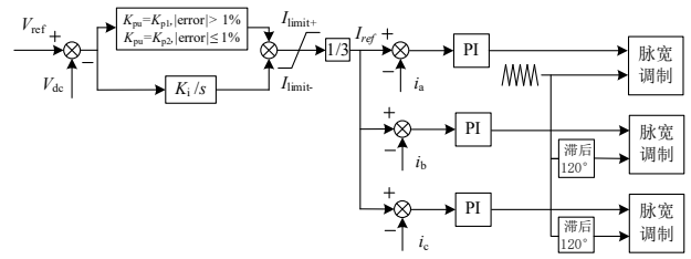
图 4 自适应双环 PI 控制框图 Fig.4 An adaptive double loop PI controller.
