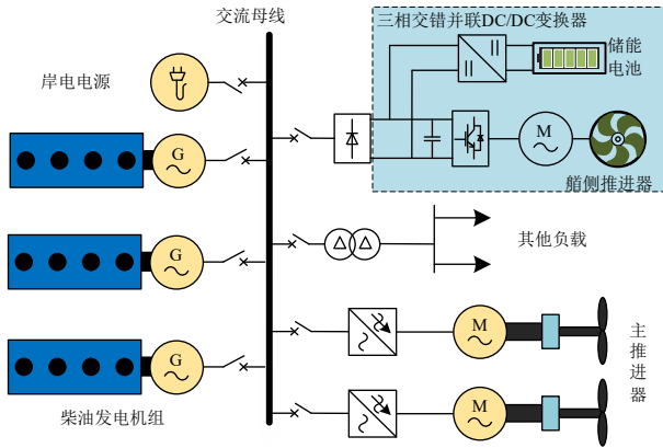
图 2 船舶微电网结构 Fig.2 Structure of shipboard microgrid.
