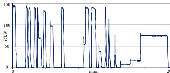
图 1 艏侧推进器功率需求 Fig.1 Power demand of bow thruster.
