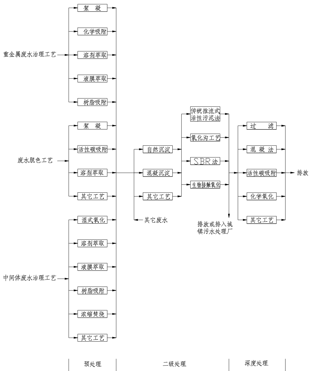
图 1 染料工业废水治理工程工艺流程图
