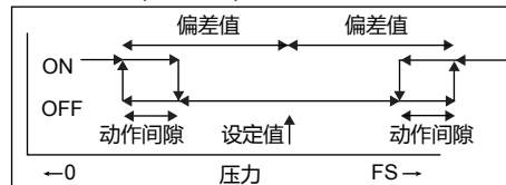
偏差上下限 (正动作)
