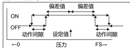
偏差上下限 (逆动作)
