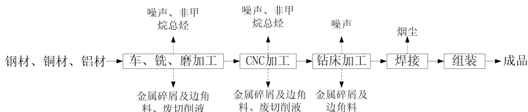
图 5-1 本项目工艺流程及产污环节图
