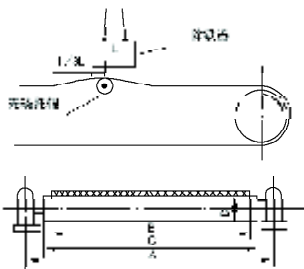
外形尺寸图
