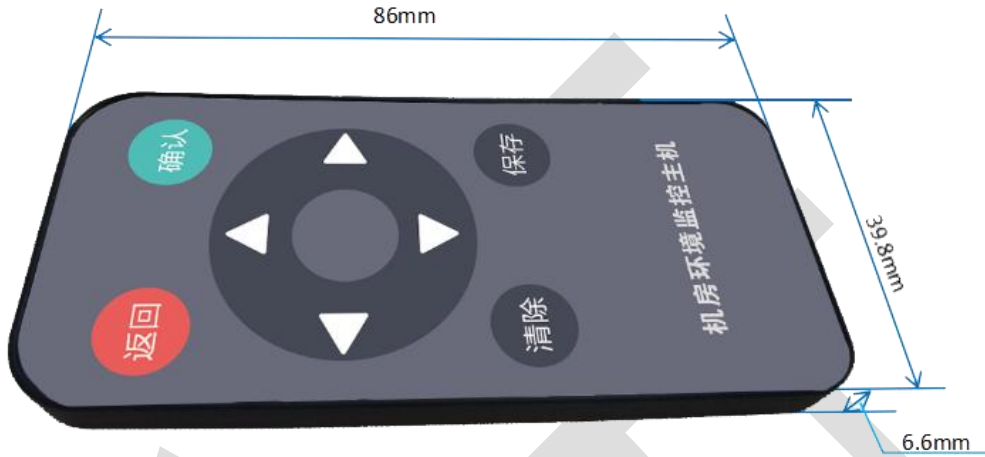
遥控器尺寸图:
