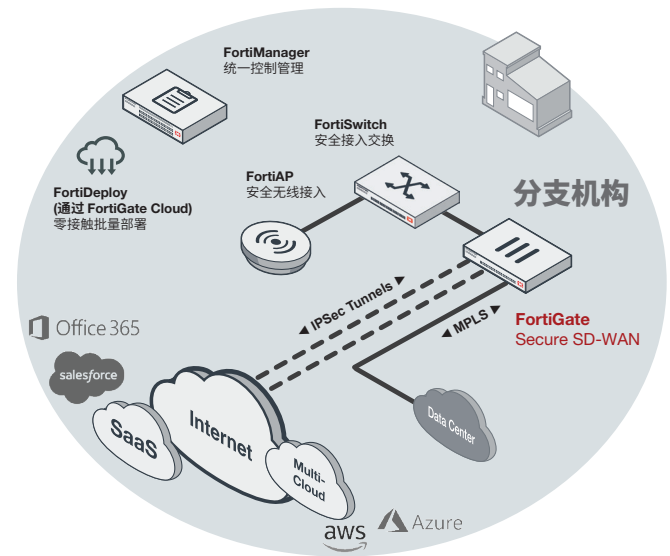
FortiGate 500E 部署在分支机构中 (安全 SD-WAN)
