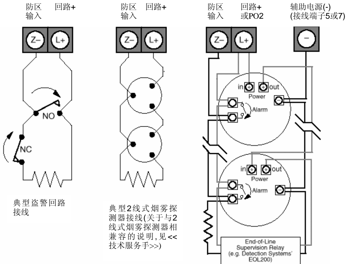
典型4线式烟雾探测器接线举例: 用一个MB4W底座的博世公司DS250烟雾探测器.
