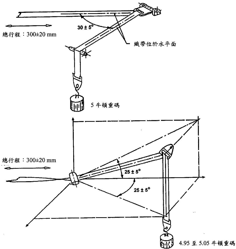
圖四 耐磨耗性試驗二
