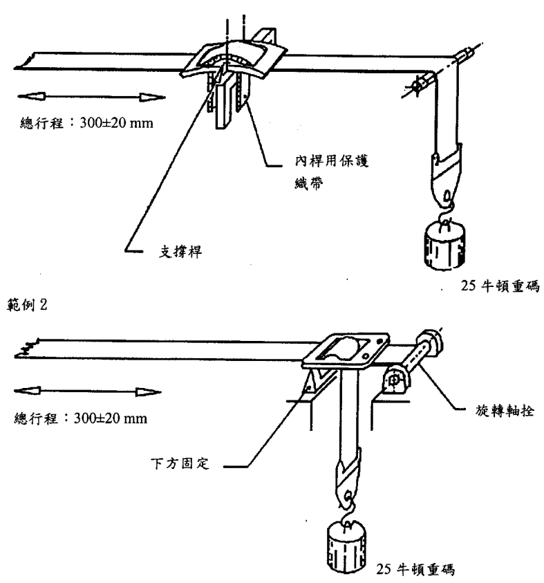
圖三 耐磨耗性試驗一
