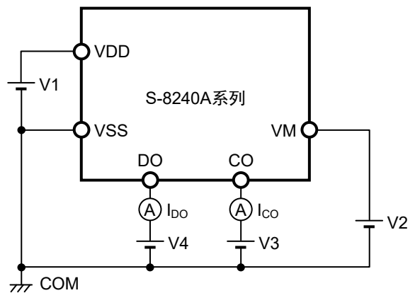
图9 测定电路4
