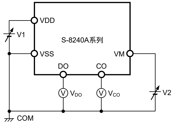
图7 测定电路2
