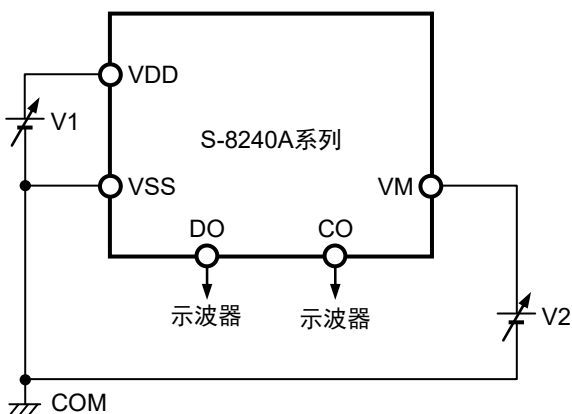
图10 测定电路5
