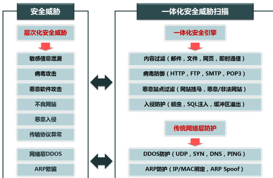
图 7 一体化安全引擎
