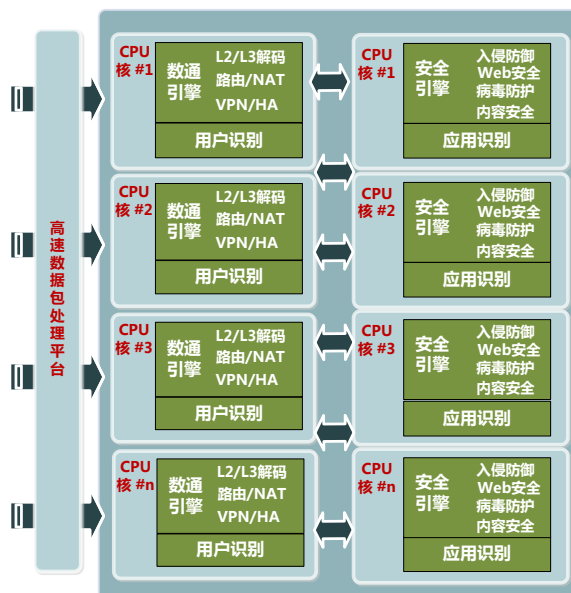
图 8 双引擎多核并发
