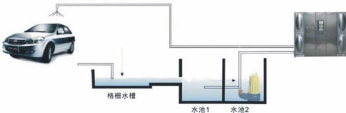
洗车水循环净化机运行流程图
