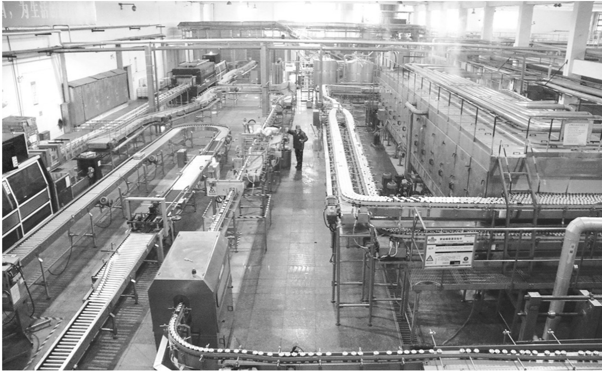
青岛啤酒易拉罐生产线
