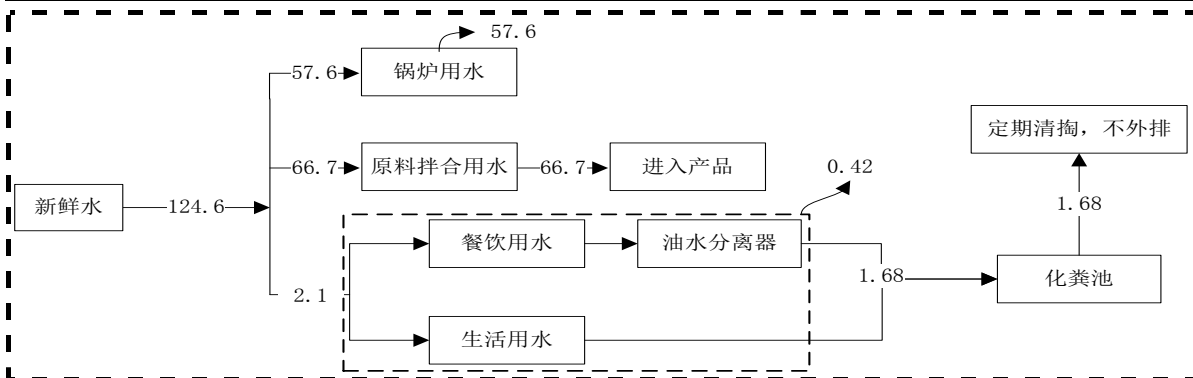
图 1 本项目用水平衡图 m 3 /d
