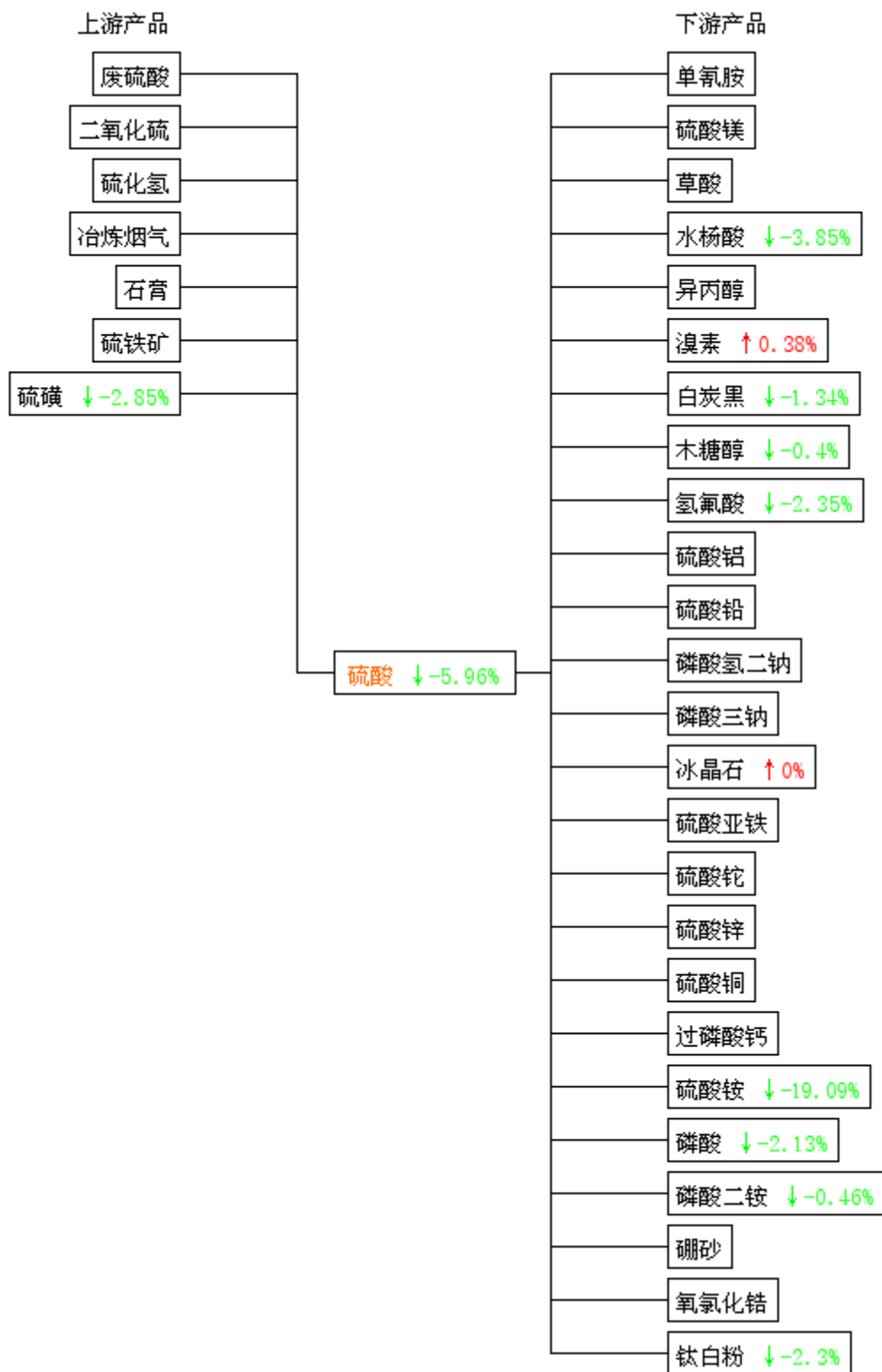
生意社硫酸产业链价格涨跌图 2012-07-01 - 2012-07-31
