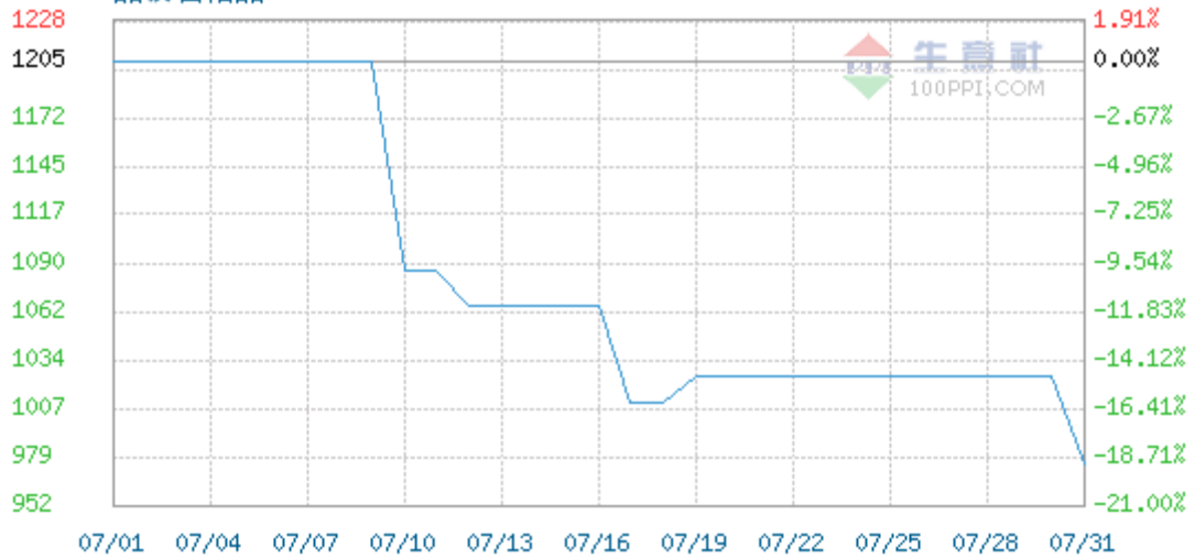
硫酸铵 国内 生产者价格 2012-07-01 - 2012-07-31
