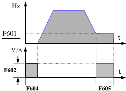
图5-11 直流制动
