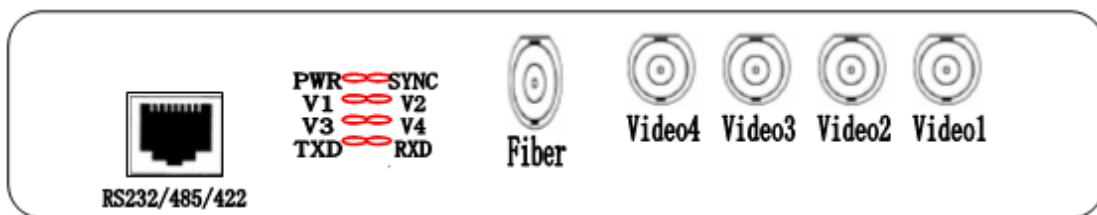
图2. 台式设备前面板图
