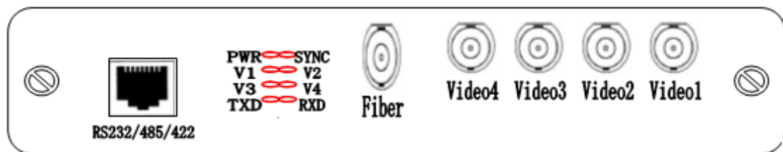
图3. 机架式设备前面板图
