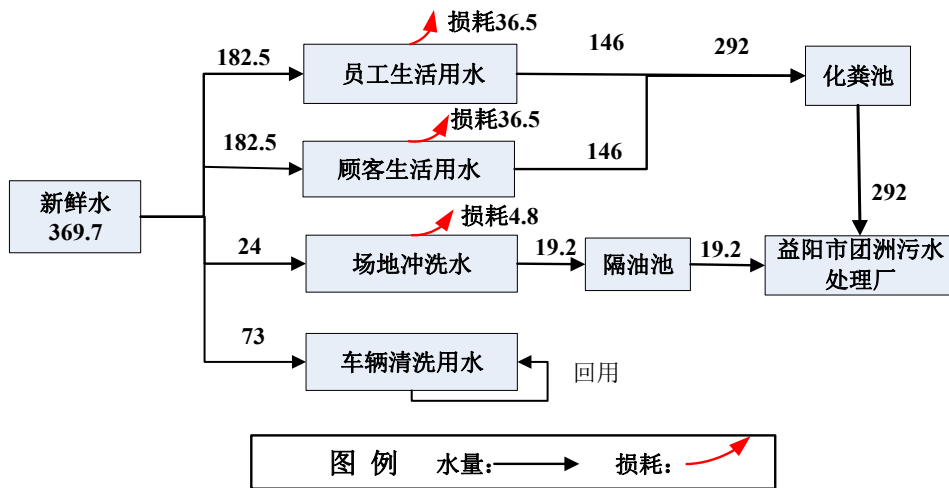
图 2-1 赫山加油站水平衡图 (m 3 /a)
