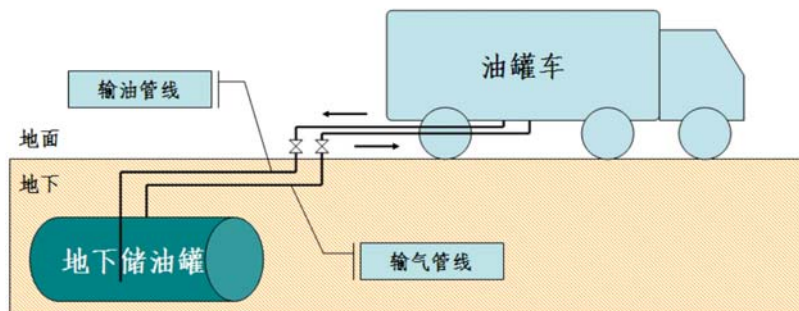
图 3-1 卸油区油气回收（一次油气回收）系统基本原理图
