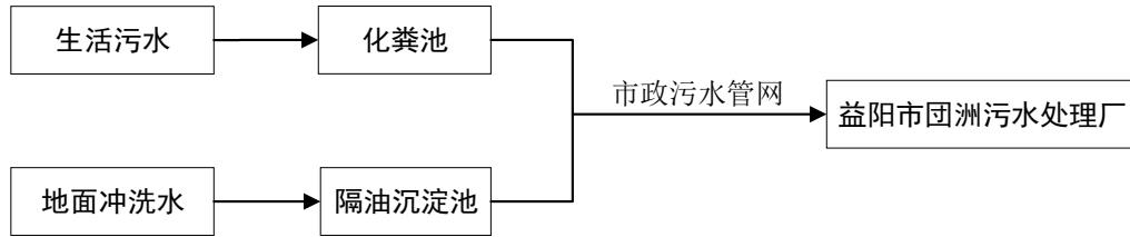
图 3-4 项目污水排放流程图
