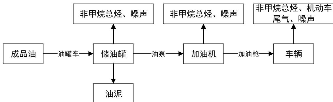
图 2-2 加油站工艺流程及产污环节图
