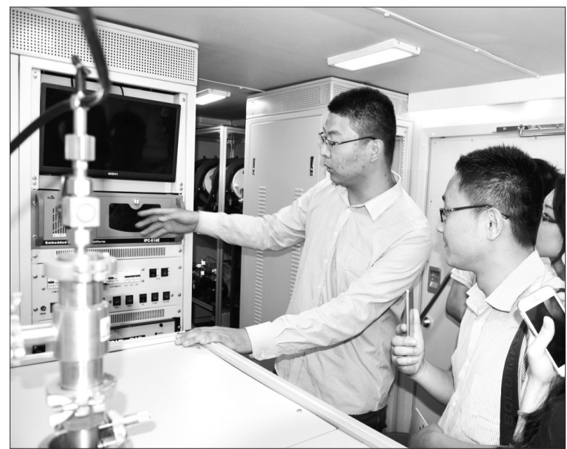
为扩大公众环境知情权,激发公众参与环保的热情,济南市环保局组织开展了“公众开放日”活动,邀请群众参观市环境监测中心站。图为工作人员向群众讲解环境在线监测设备。 卞胜军摄
