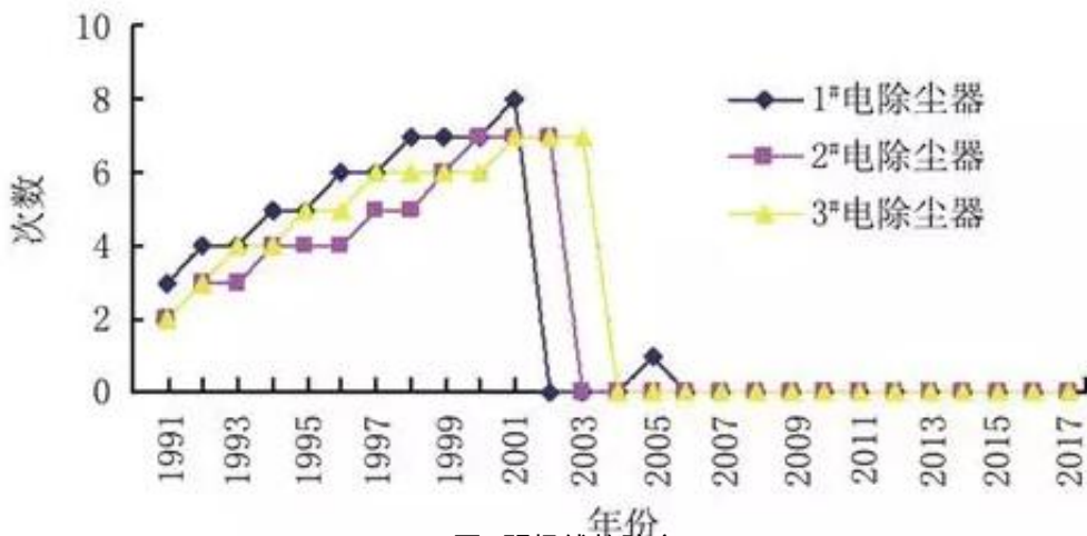
图2 阴极线故障率
