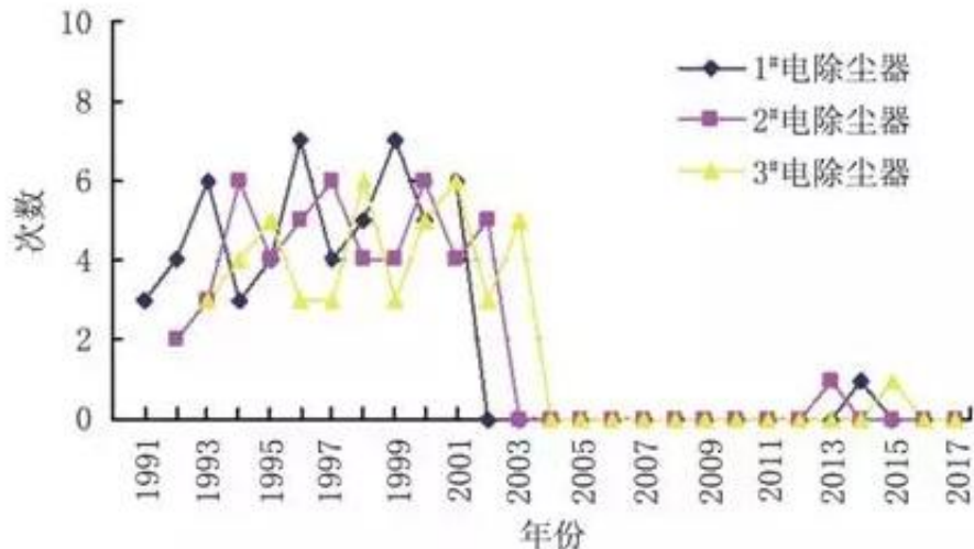
图1 尘中轴承故障率
