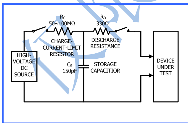
图10a. IEC 61000-4-2 ESD测试模型
