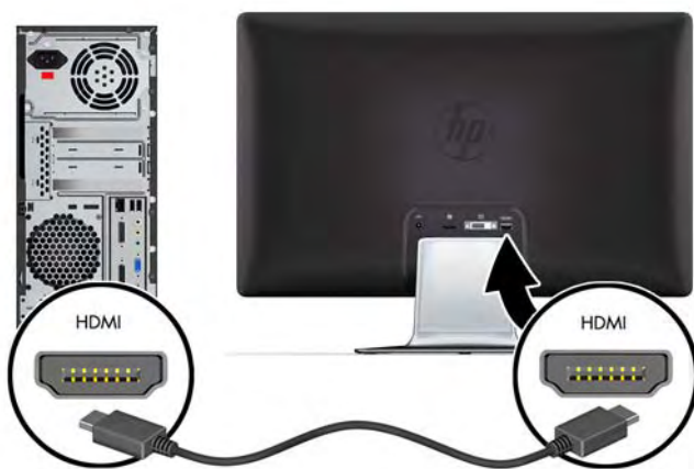
图 3-5 正在连接 HDMI 电缆（只在选定型号提供此电缆）
