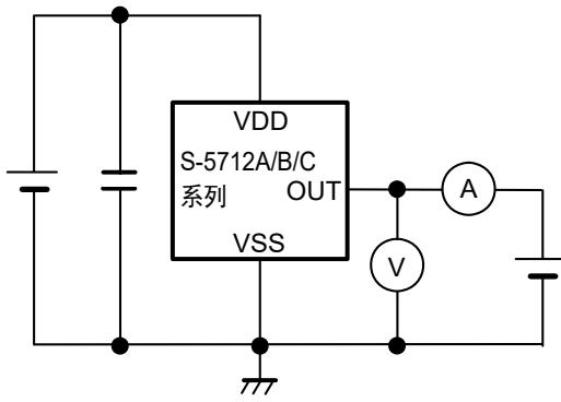
图8 测定电路4
