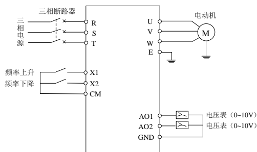
图 9-4 基本接线图
