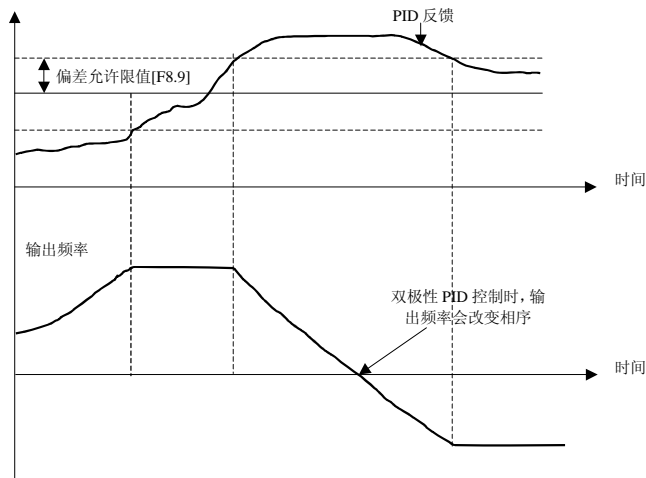
图 6-31 双极性 PID 控制方式
