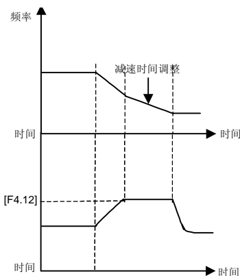
图 6-20 加速力矩与制动力矩示意图
