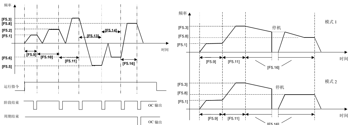
图 6-24 PLC 断点恢复
