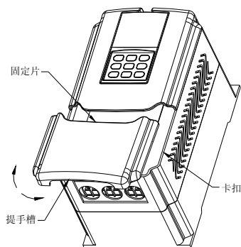
图 2-3-A 塑壳盖板的拆卸与安装
