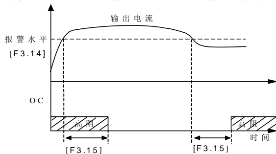
图 6-16 过载报警
