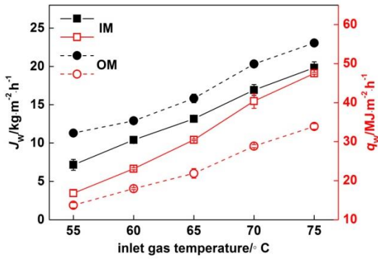
图 6 进气温度对水通量和热通量的影响
