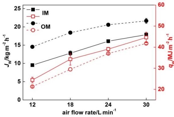
图 4 进气流量对水通量和热通量的影响
