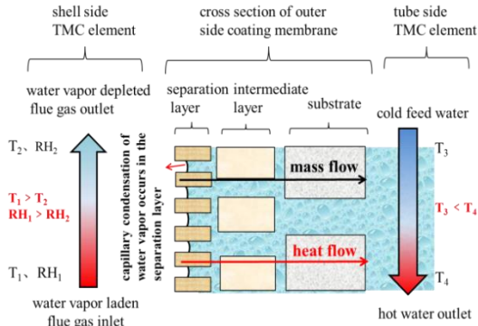
图 2 陶瓷外膜冷凝器的 TMC 过程示意图
