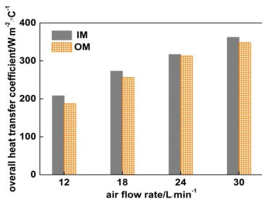
图8 陶瓷内膜和外膜总传热系数的比较
