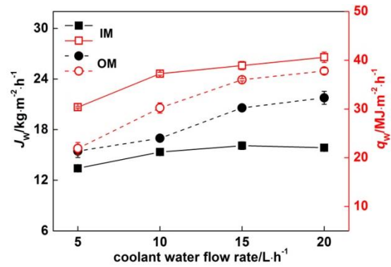
图 5 冷却水流量对水通量和热通量的影响
