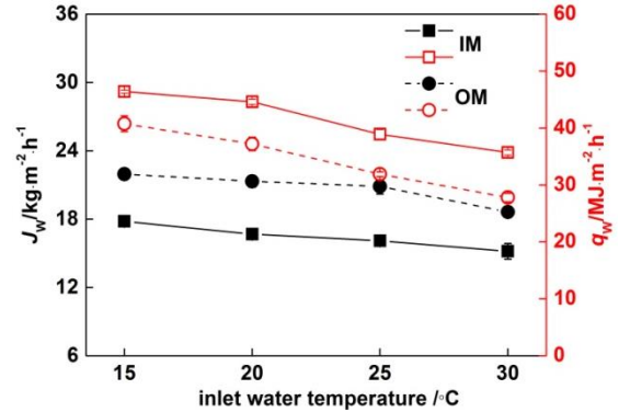
图 7 冷却水温度对水通量和热通量的影响
