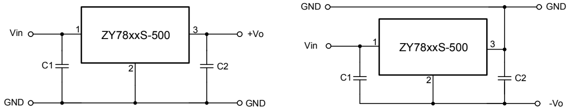
图 1 正输出（左）和负输出（右）应用电路图
