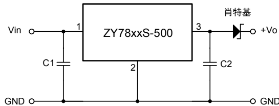
图 2 保护电路
