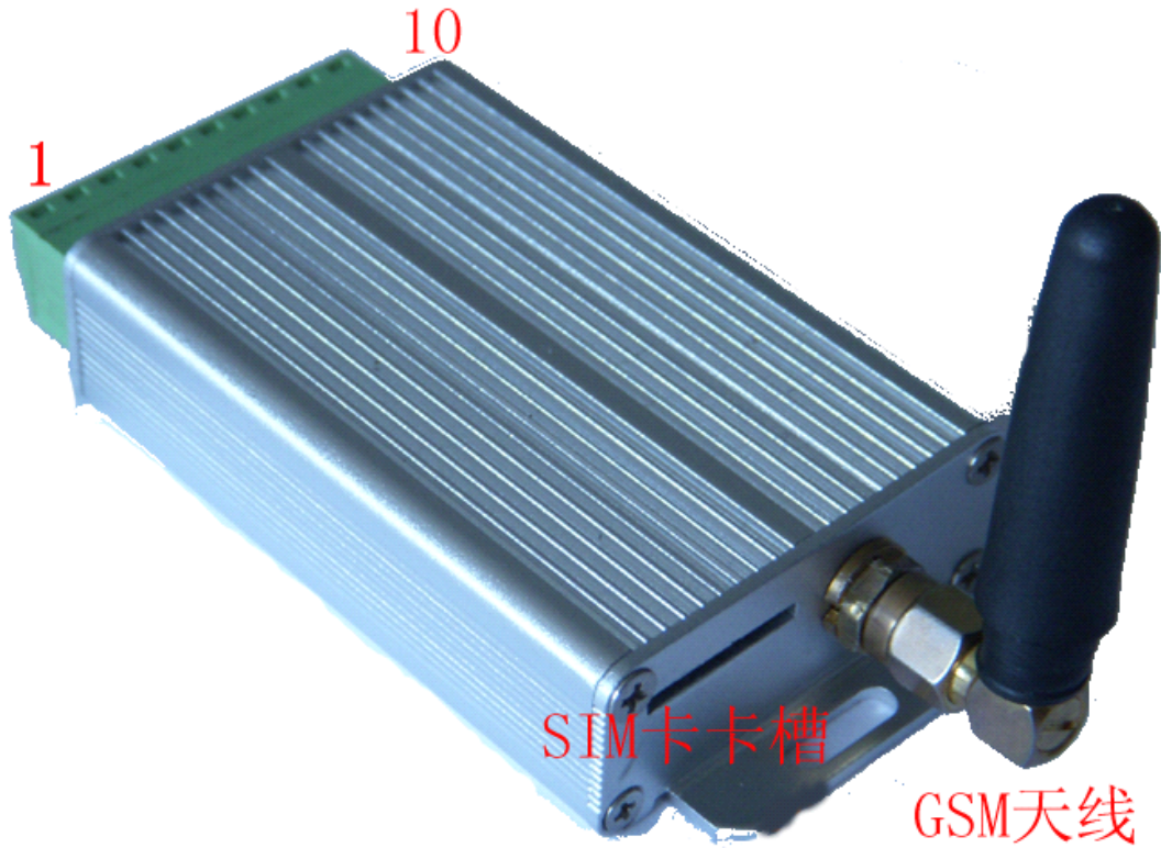
图 3-2 DTU-C 实物图
