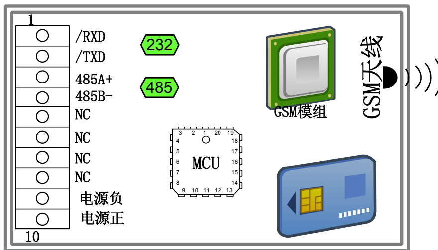
图 3-3 DTU-C 内部功能结构图
