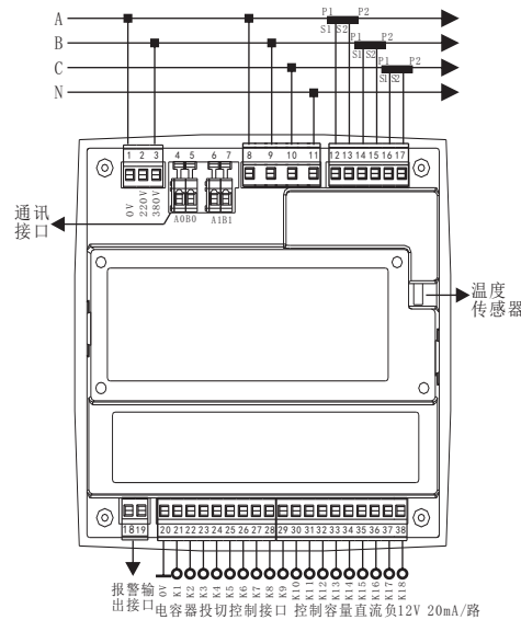
JKW-15FA-18D型控制器接线图(动态输出)电源取380V
