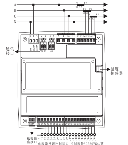
JKW-15FA-18J型控制器接线图(静态输出)电源取220V
