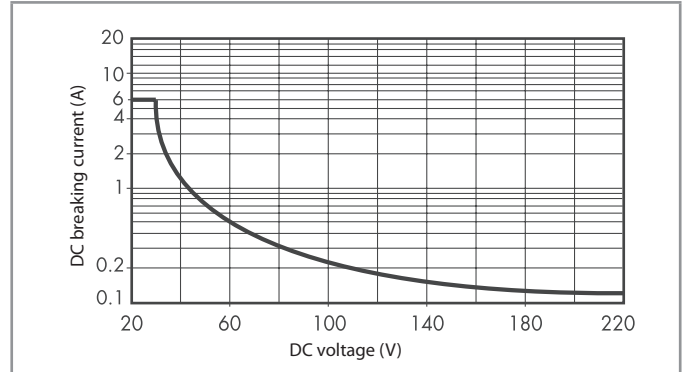
H 34 - 最大DC斷流容量
