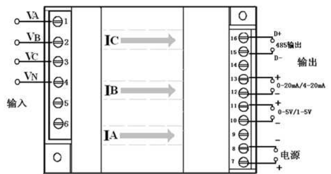
图 4: CE-AJ41-3**DS5 三相四线接线图
