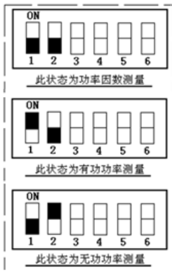
图 5 测量功能设置
