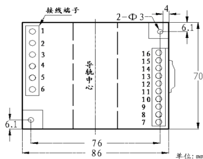
图 2. 导轨安装尺寸图
