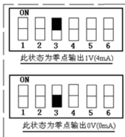
图 6 零点输出设置
