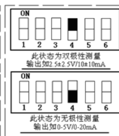
图 7 极性测量设置
