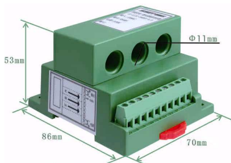
图 1. CE-AJ41-3**DS5 产品外观图
