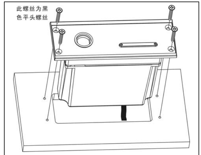
图 3.53 HCS-4841NC/20、HCS-4341ND/20 及 HCS-4842N/20 单元安装图
