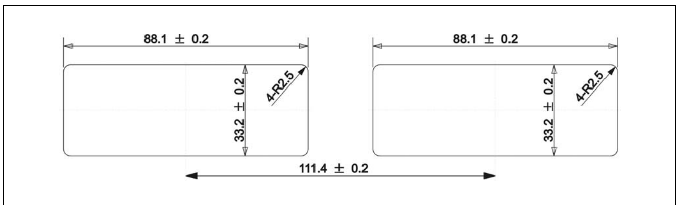
图 3.54 N 系列会议单元组合式安装定位图
