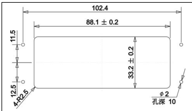
图 3.52 HCS-4841NC/20、HCS-4341ND/20 及 HCS-4842N/20 单元开孔定位图（单位：mm）
