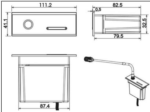
图 3.51 HCS-4841NC/20、HCS-4341ND/20 及 HCS-4842N/20 单元外形尺寸图（单位：mm）
