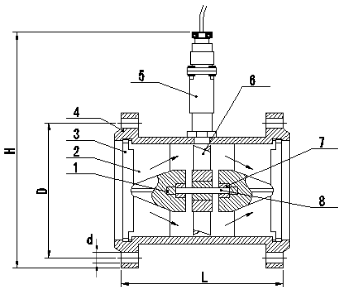
图（二） LWGY—15~40 传感器结构及安装尺寸示意图
