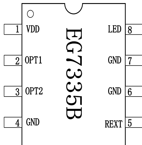
图 4-2. EG7335B SOP8 管脚定义
