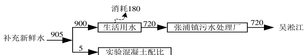
图 5-3 项目水平衡图 (t/a)
