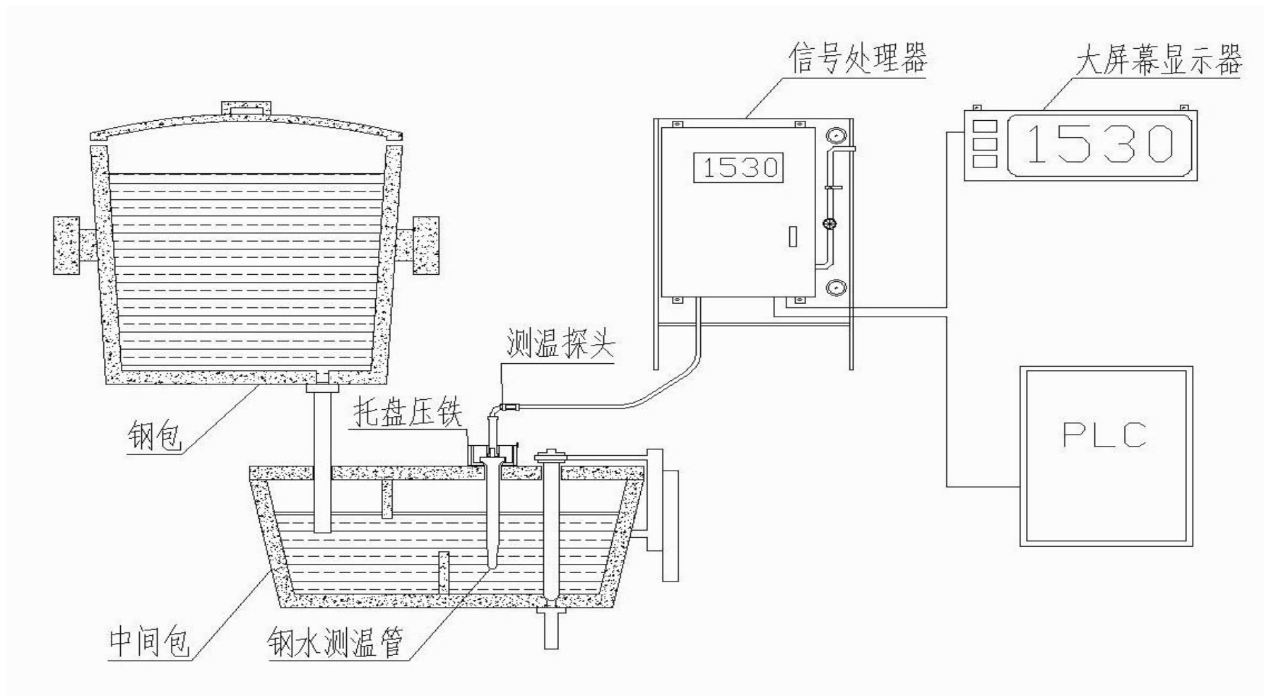
安装示意图 2:
