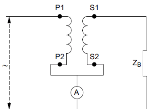
图 2D.4 1:1 电流互感器的基本电路
