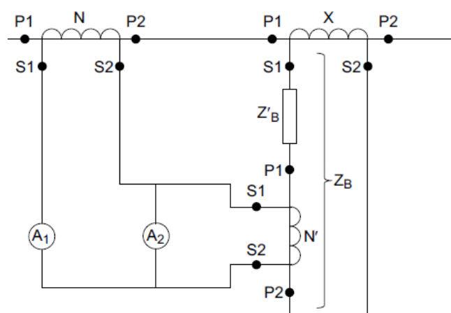
图 2D.6 另一种试验电路
