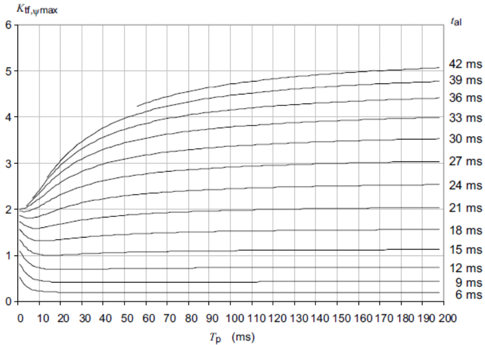
图 2E.6 K_{tf} 的确定 (在时间范围 1 及 16.7 Hz 和 T_s = 5.5s 条件下)
