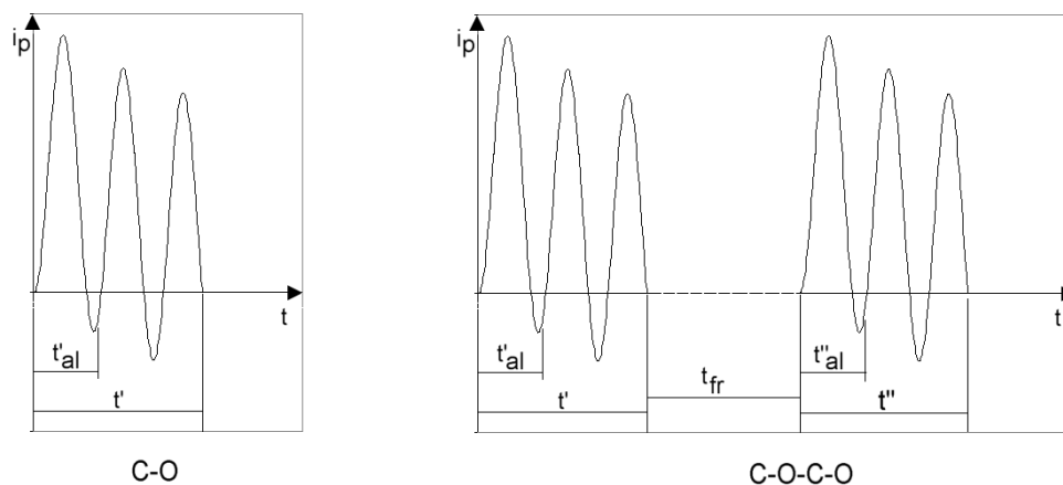
图 201 工作循环
