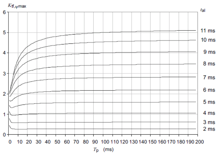
图 2E.5 K_{tf} 的确定 (在时间范围 1 及 60 Hz 和 T_s = 1.5s 条件下)
