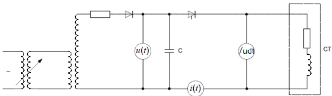
图 2E.13 电容放电法的电路
