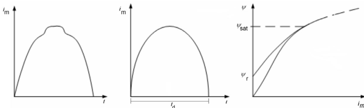
图 2E.14 电容放电法的典型记录图
