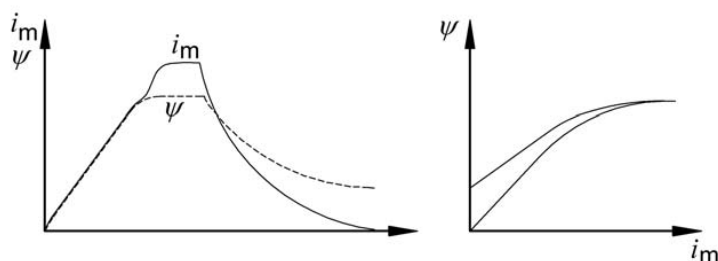
图 2E.11 时间与幅值及磁通与电流的图形
