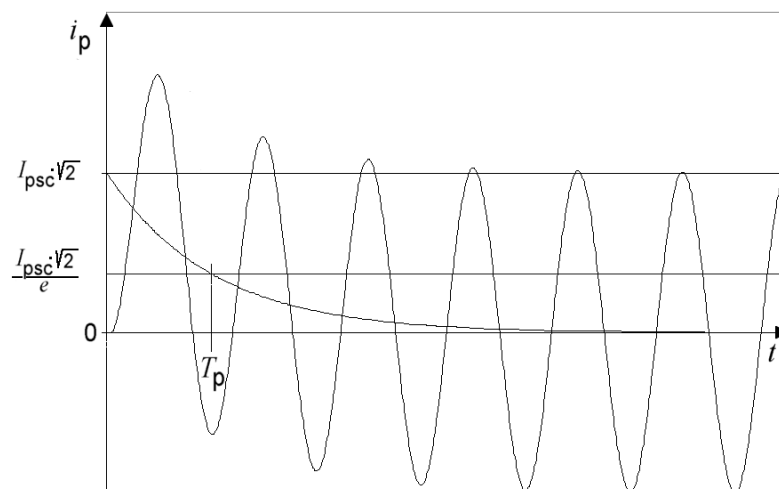
图 202 一次时间常数 T_p
