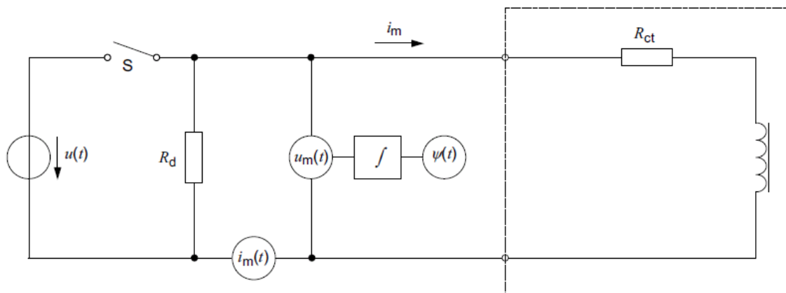
图 2E.10 直流法的电路
