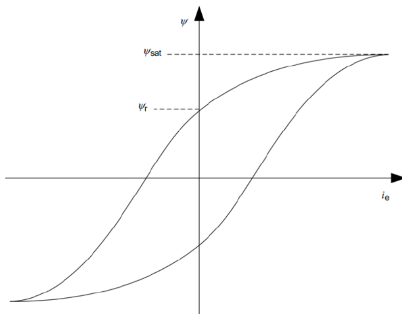
图 2E.9 磁滞回环确定剩磁系数
