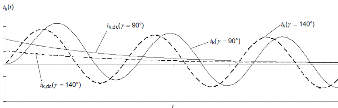
图 2E.1 两种故障初始角的短路电流
