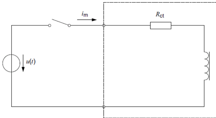
图 2E.8 基本电路
