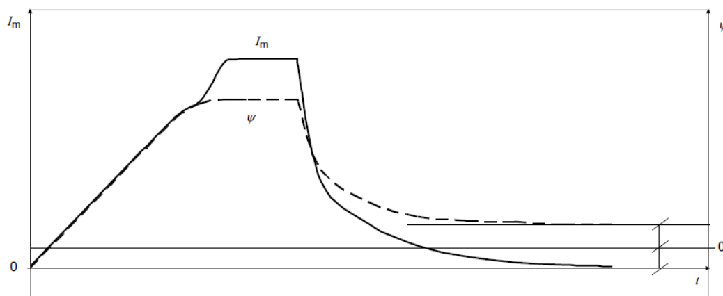
图 2E.12 磁通基线平移的记录图
