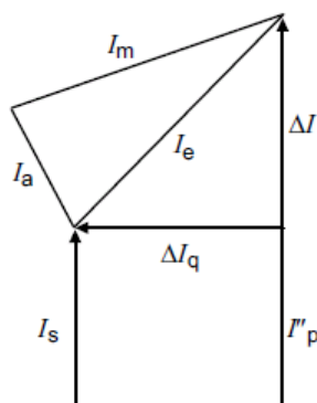
图 2D.2 误差三角形
