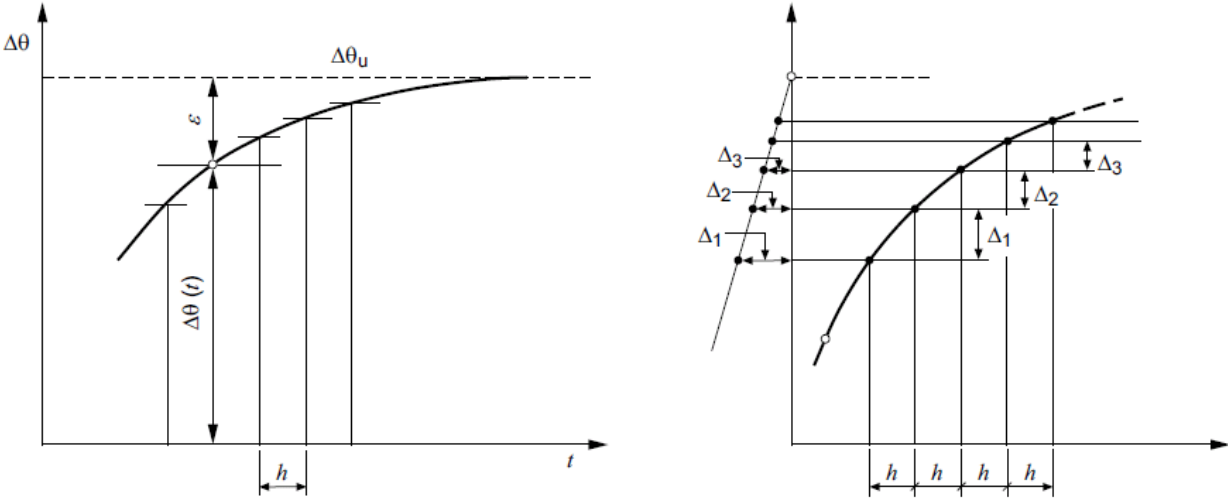
图 2F.1 估算最终温升的外推图
