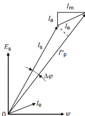
图 2D.1 相量图
