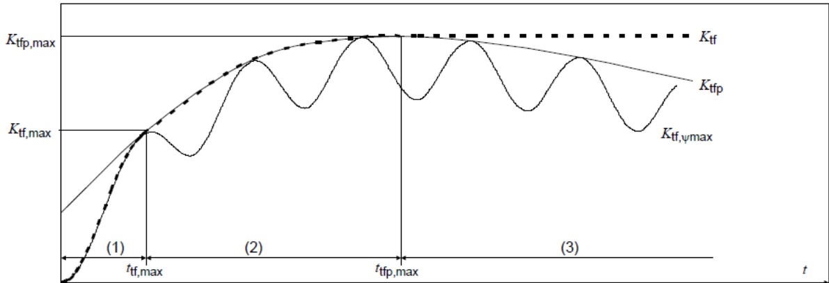
图 2E.3 暂态系数计算的有关时间范围
