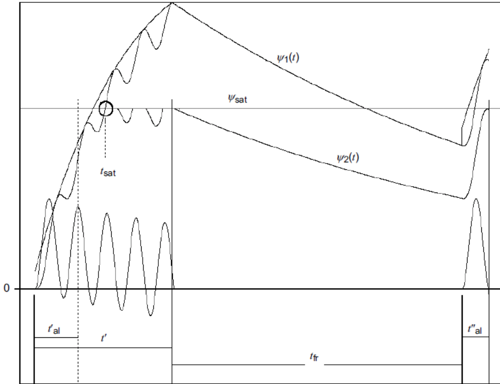
图 2E.7 铁心饱和对磁通的限制
