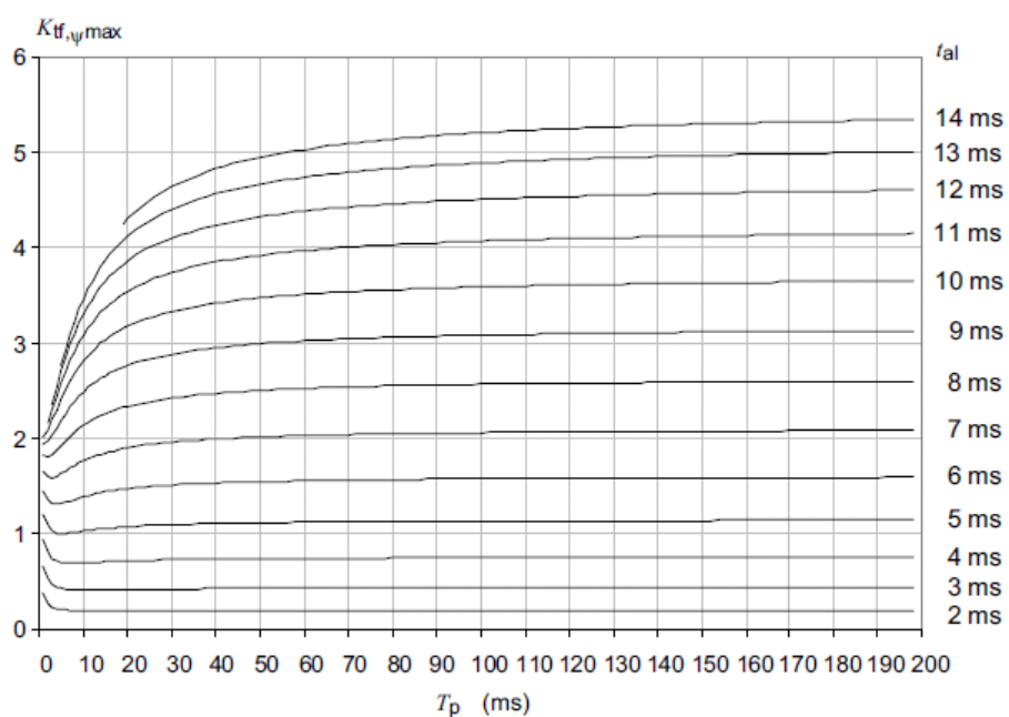
图 2E.4 K_{tf} 的确定 (在时间范围 1 及 50 Hz 和 T_s = 1.8s 条件下)
