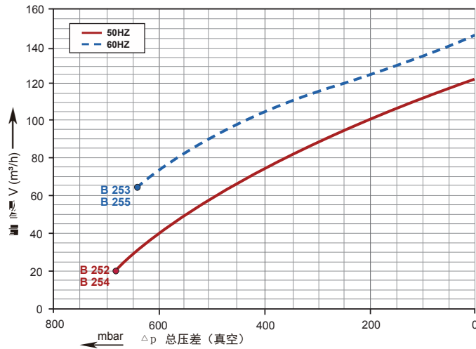
真空性能曲线
