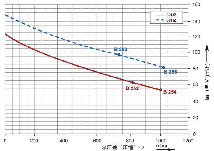
压力性能曲线
