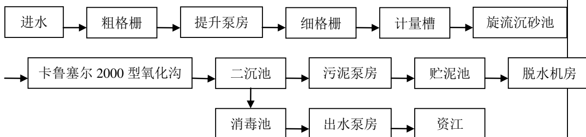
图 1 城北污水处理厂污水处理工艺流程图
