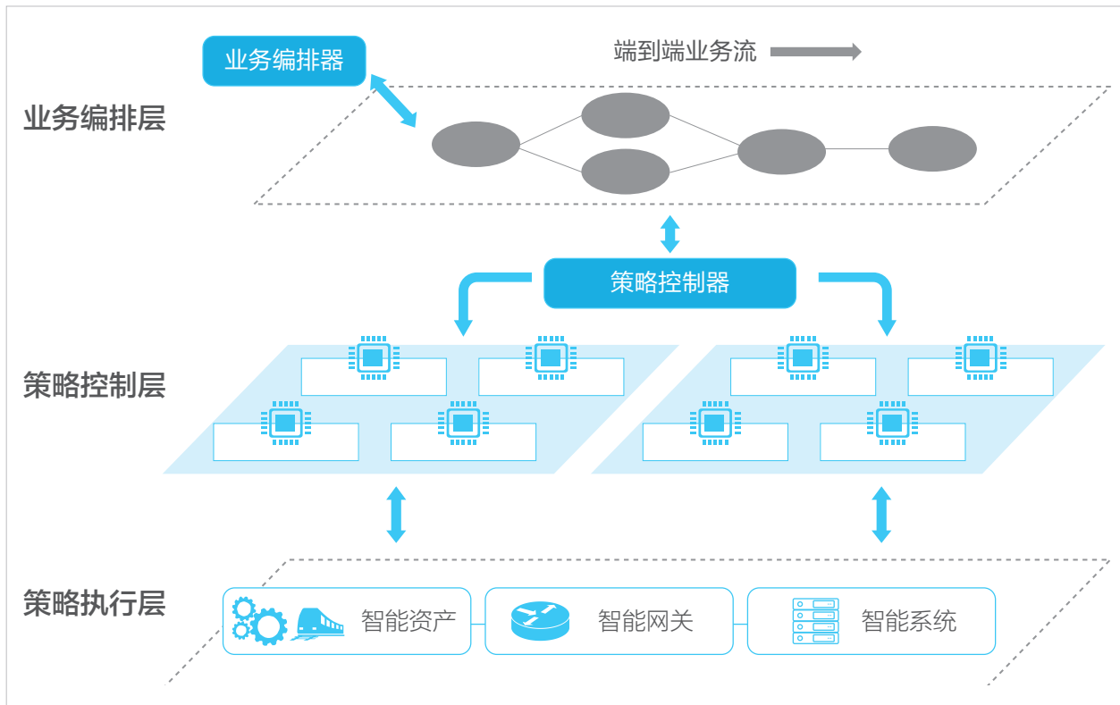
图12 功能视图：业务编排分层
